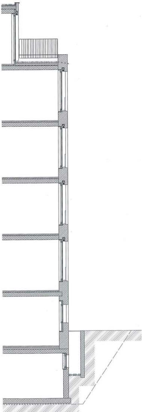
Fassadenschnitt
